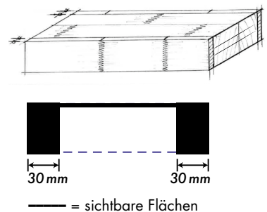
tr optina Futter II 3-seitig sichtbar
