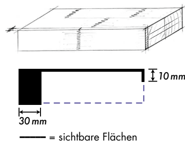
tr optina Futter I 2-seitig sichtbar
