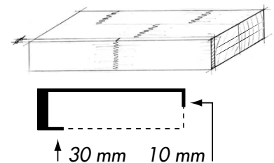
tr optina Futter I 2-seitig sichtbar
