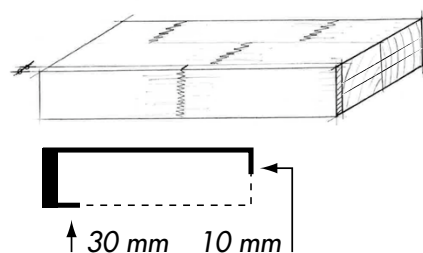
tr optina Futter I 2-seitig sichtbar
