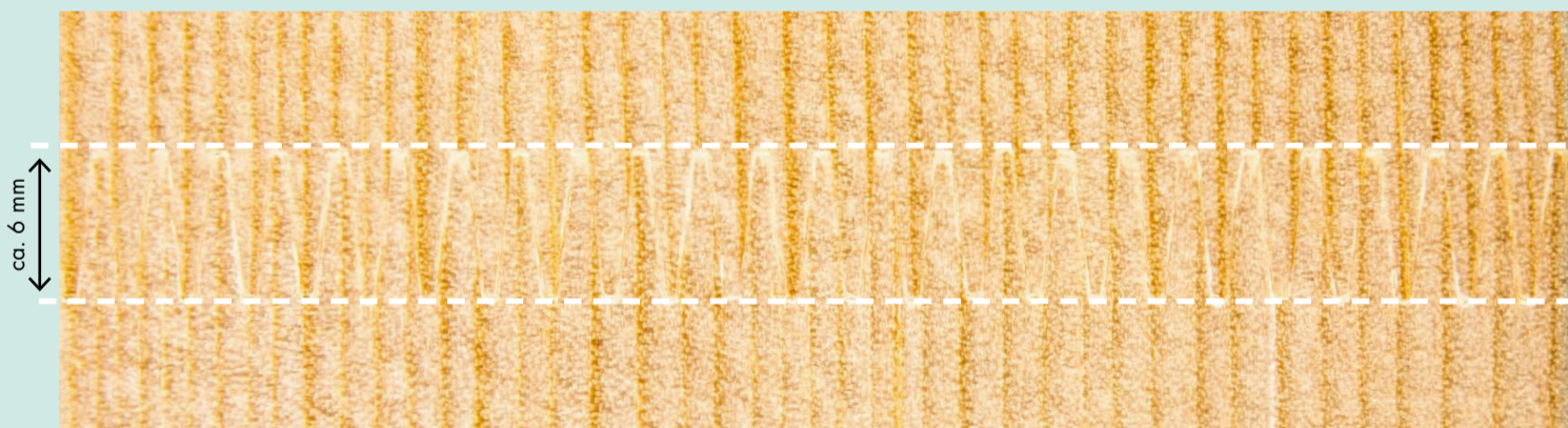
Keilzinkenverbindungen neu (Ansicht vergrössert)
